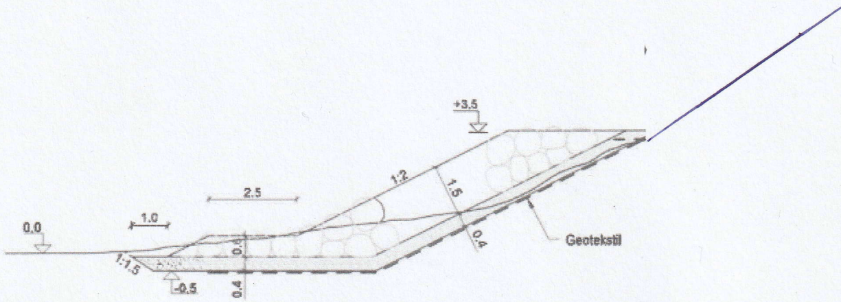
PRINCIPSNIT , 1:100
